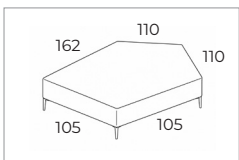
TERMINALE DX - SX RIGHT / LEFT END UNIT
